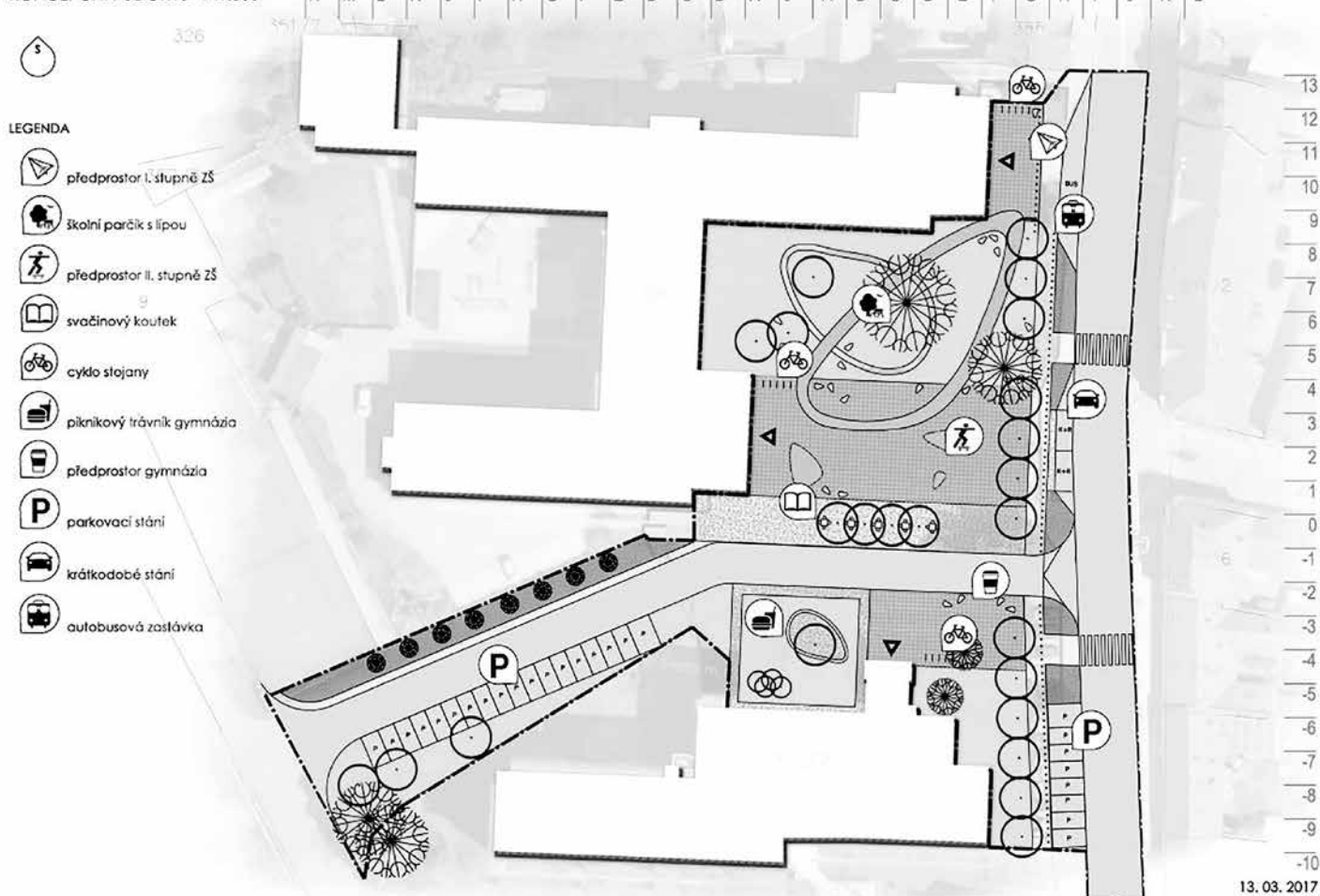
KONCEPČNÍ PŮDORYS M1:500
